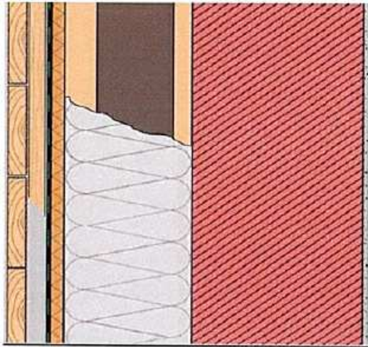
Figur 13 (ordregivers tegning)
