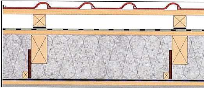
Figur 3 (ordregivers tegning)
